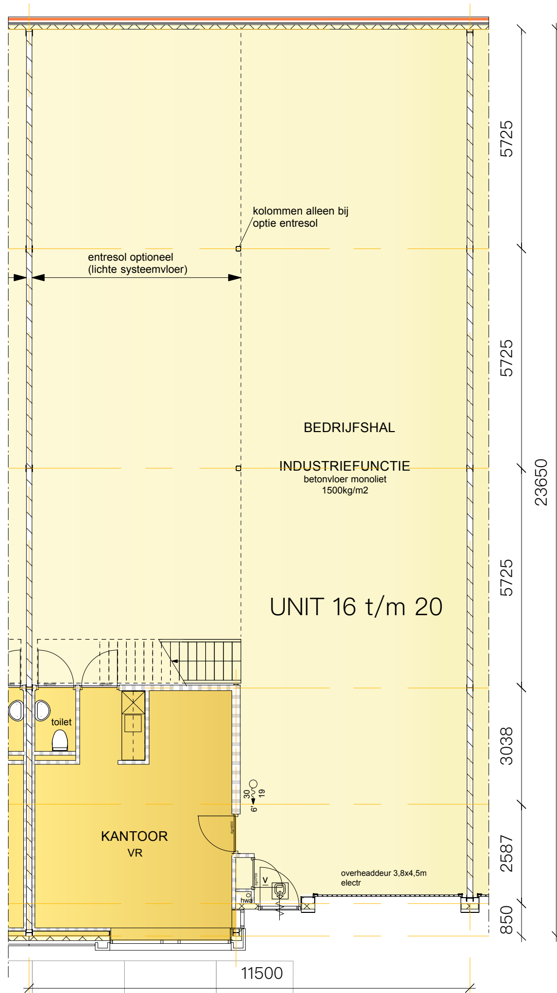
UNIT 16 t/m 20 begane grond
