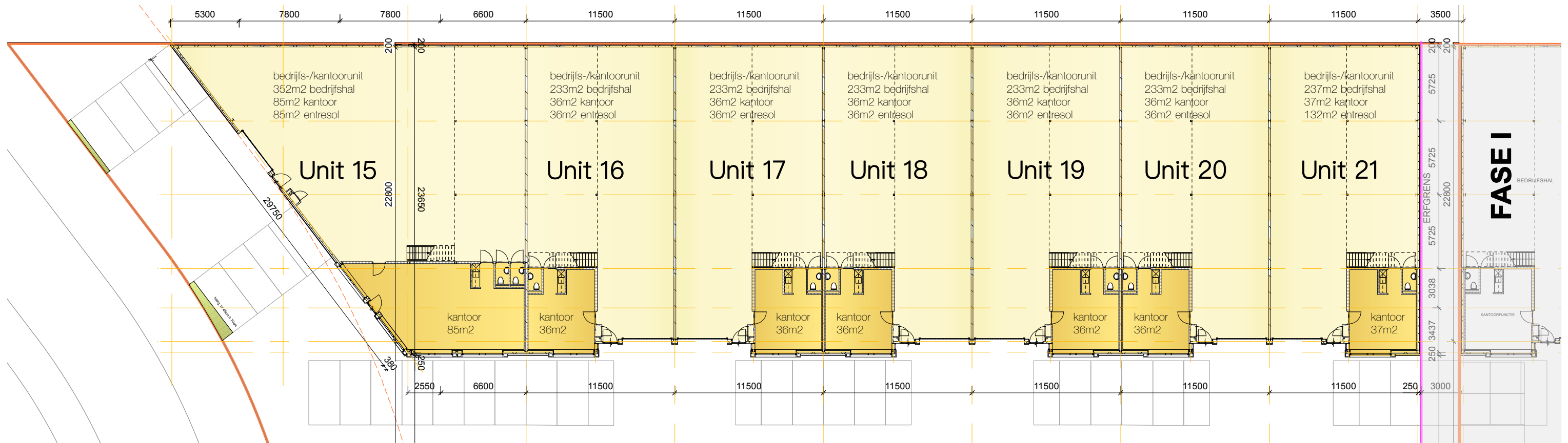
BLOK 2 BEGANE GROND
