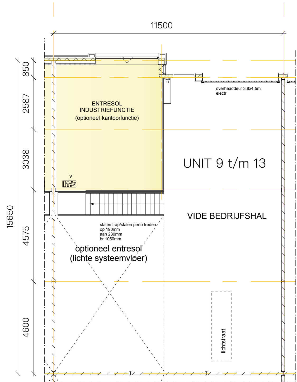
UNIT 9 t/m 13 verdieping
