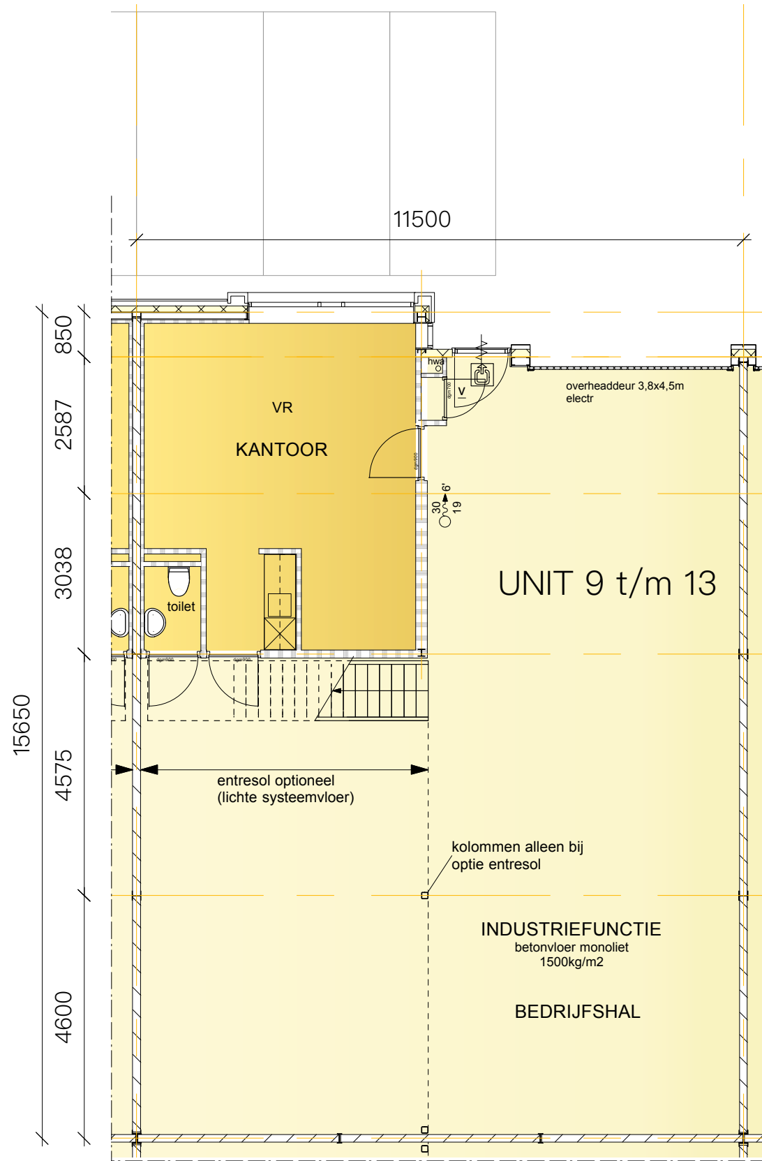
UNIT 9 t/m 13 begane grond
