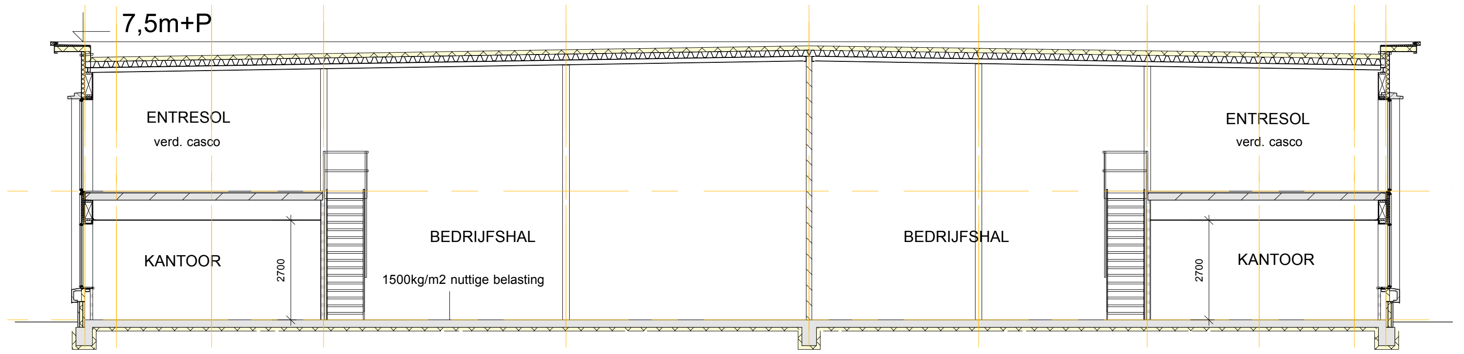
DOORSNEDE UNIT 2 t/m6 en 9 t/m13
