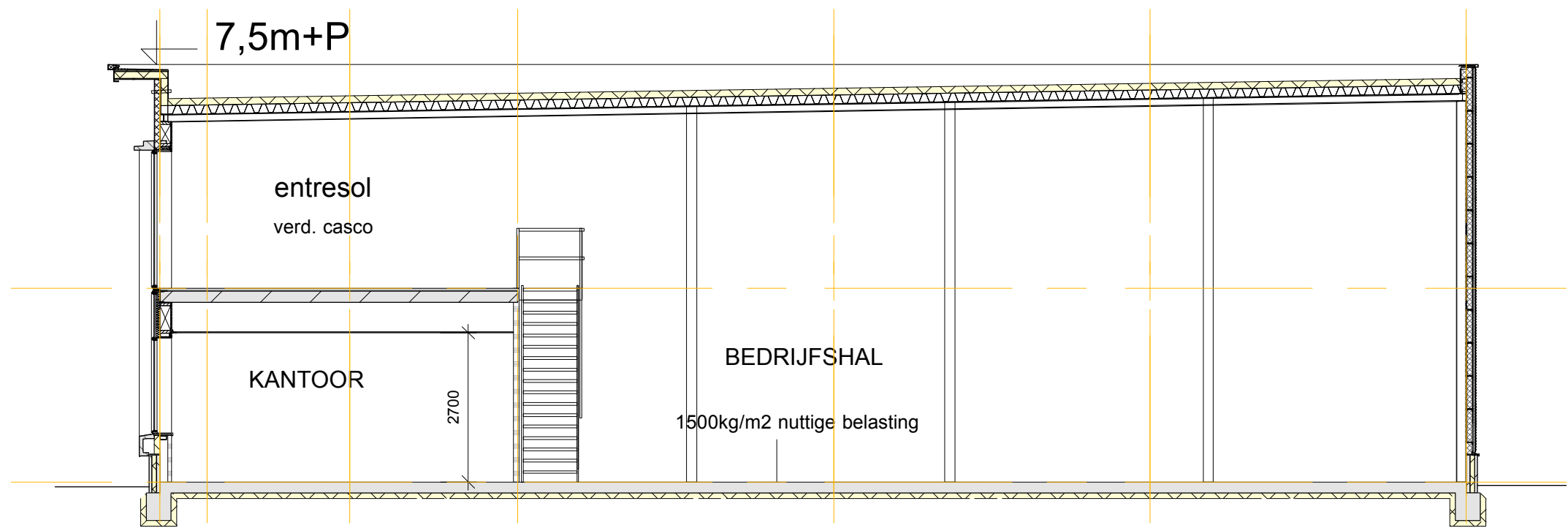
DOORSNEDE UNIT 16 t/m20
